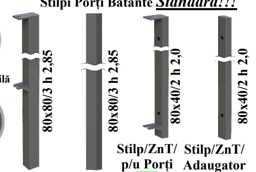
Balama Ajustabilă
